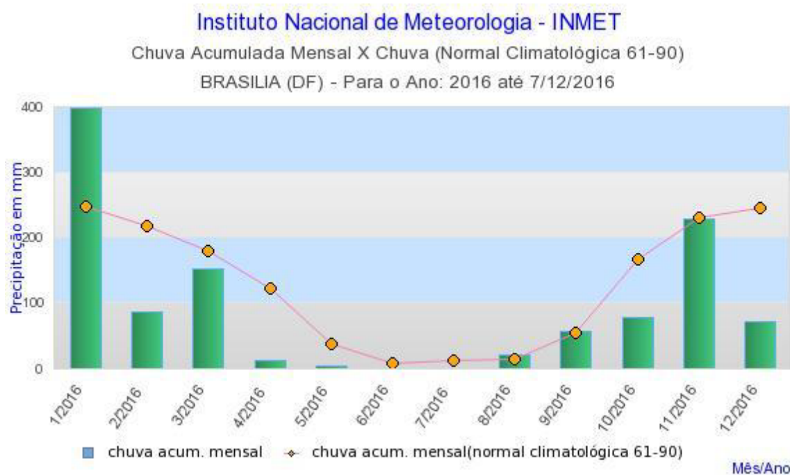
Gráfico 18 - Chuvas ocorridas X Médias Mensais
