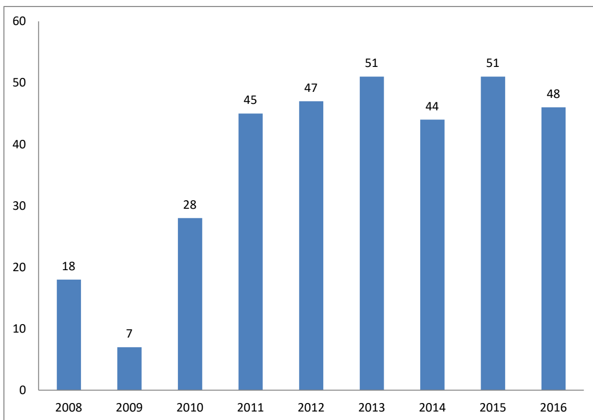
Gráfico 1. Número de parques e unidades de conservação atingidas por incêndios florestais.
