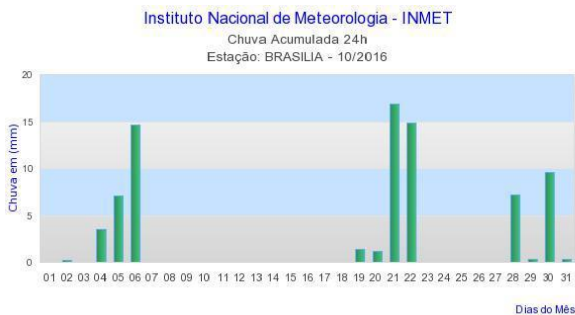
Gráfico 15 - Chuvas diárias acumuladas em outubro/2016.
